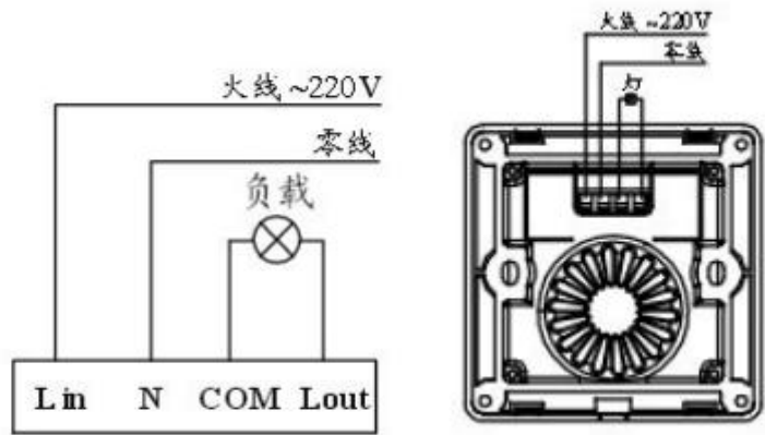
图（二）火零线声光控开关接线示意图
