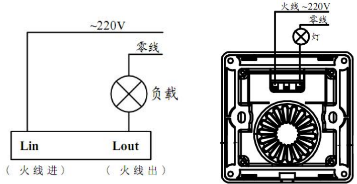
图（一）单火线声光控开关接线示意图
